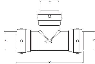
Tee
