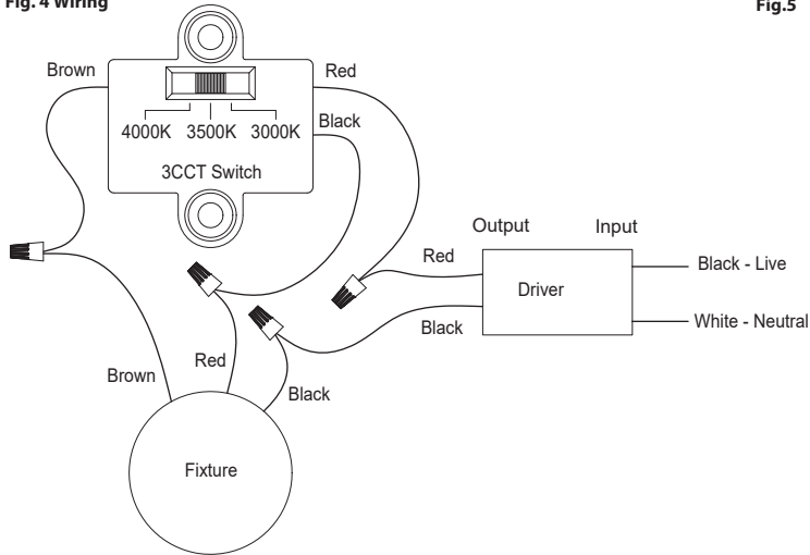
Fig. 4 Wiring
